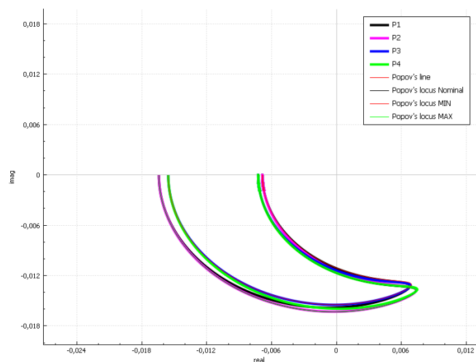
Рис. 2- Модифицированные амплитудно-фазовые характеристики исследуемой системы.
