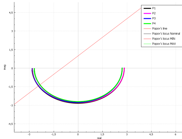
Рис. 1 - Модифицированные амплитудно-фазовые характеристики исследуемой системы.
