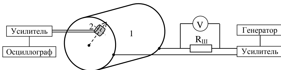
Рис. 3. Схема измерительной установки.
